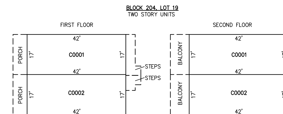
DETAILS SCALE: 1"=20'
