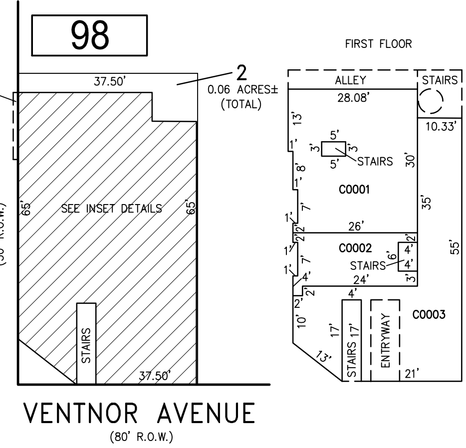
PLAN SCALE: 1"=20'
