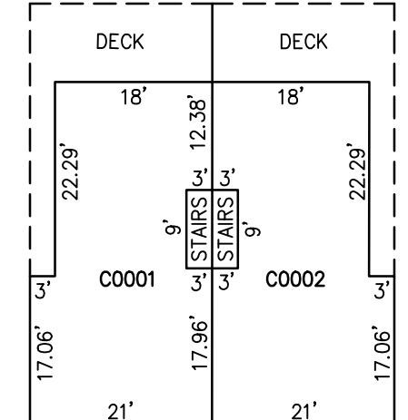
DETAILS SCALE: 1"=20'
