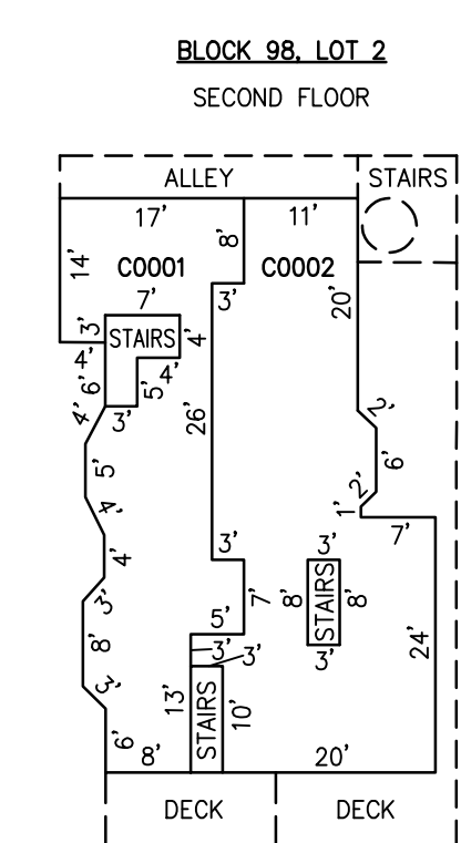
DETAILS SCALE: 1"=20'
