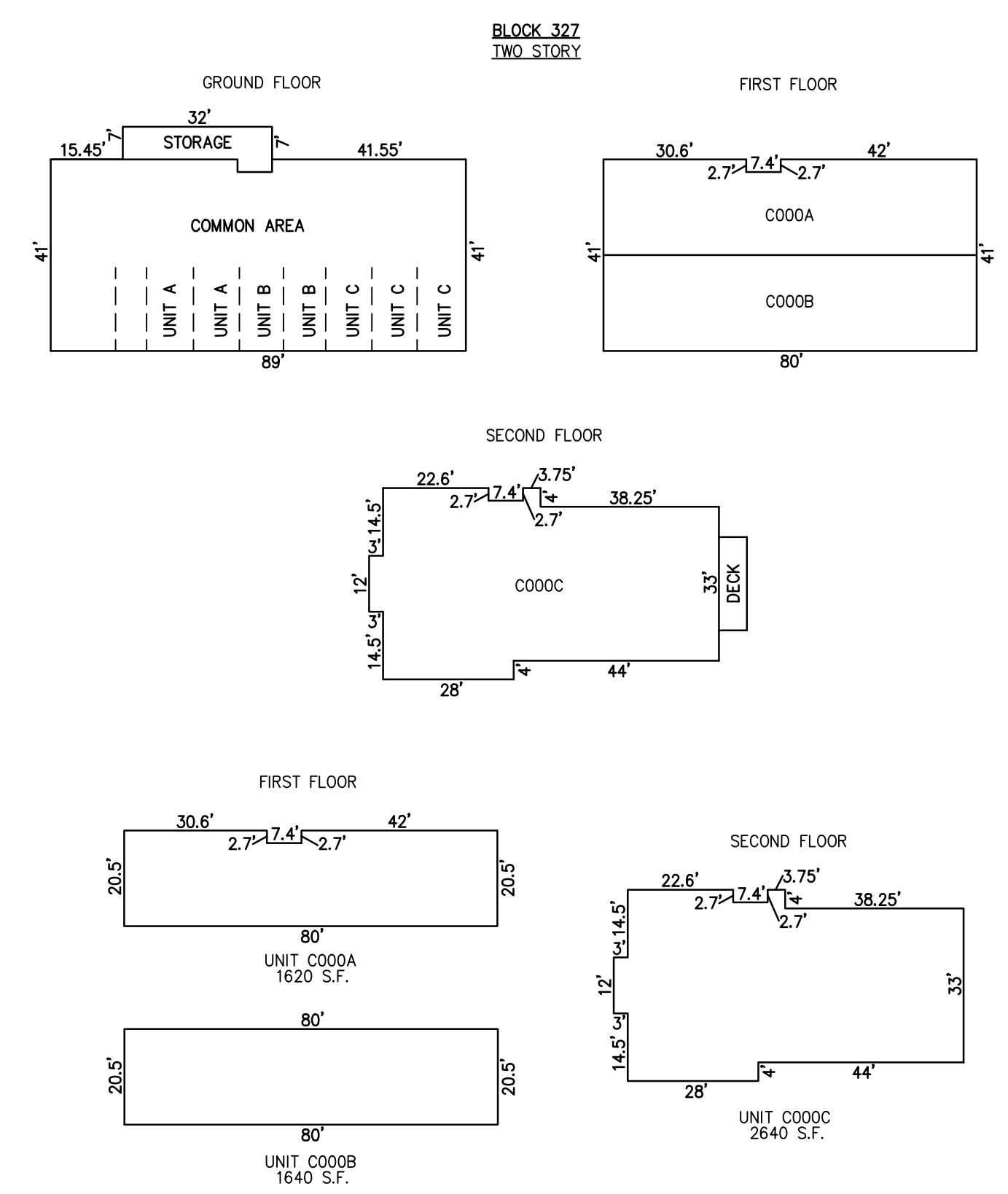
DETAILS SCALE: 1"=30"
