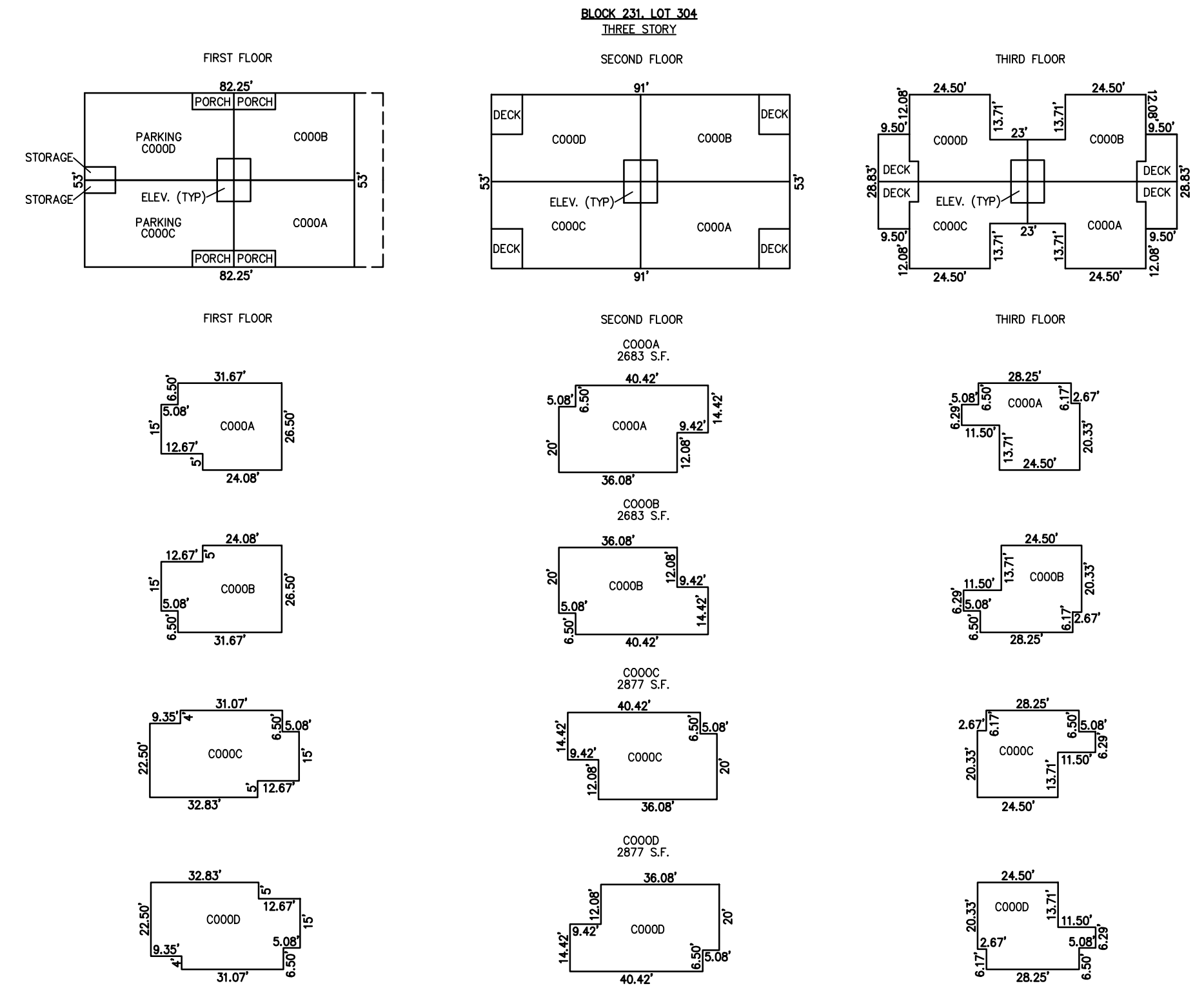
DETAILS SCALE: 1"=30"
