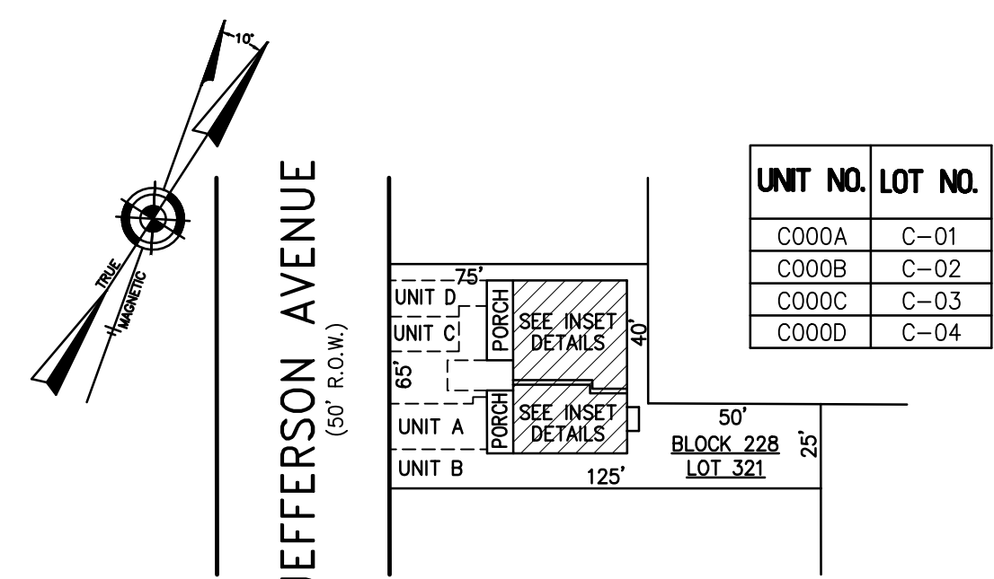
PLAN SCALE: 1"=50"
