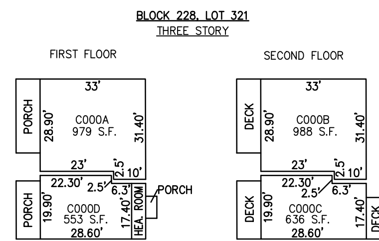
DETAILS SCALE: 1"=30"
