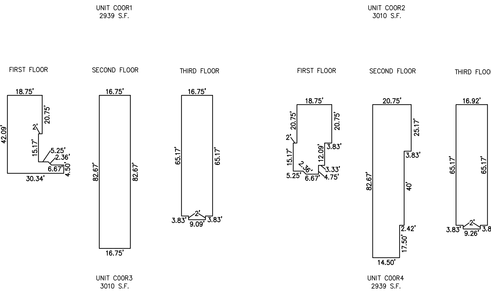
DETAILS SCALE: 1"=30'
