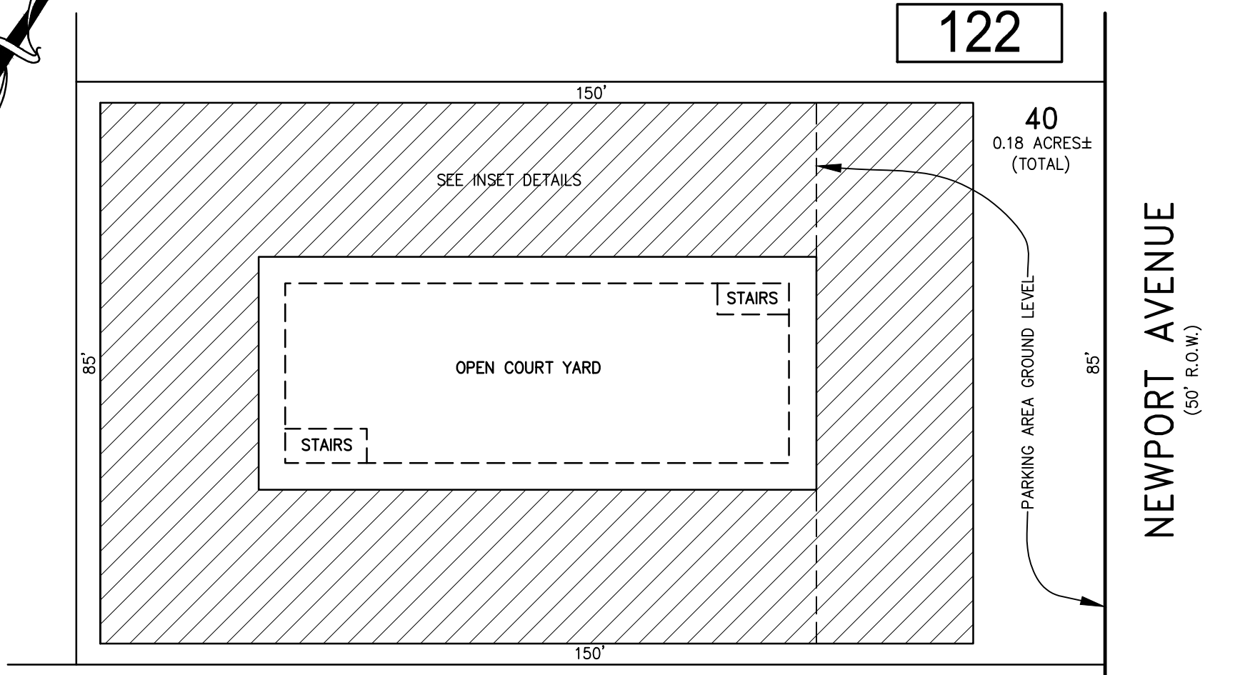
PLAN SCALE: 1"=20'
