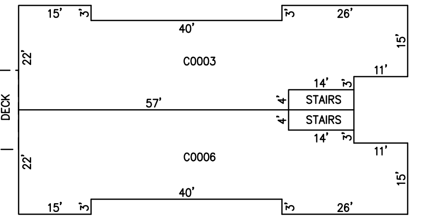
DETAILS SCALE: 1"=20'
