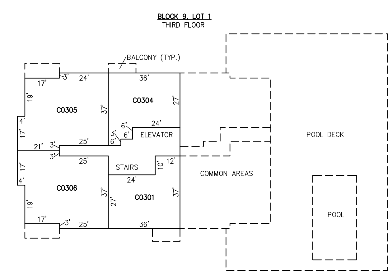
PLAN SCALE: 1"=30'
