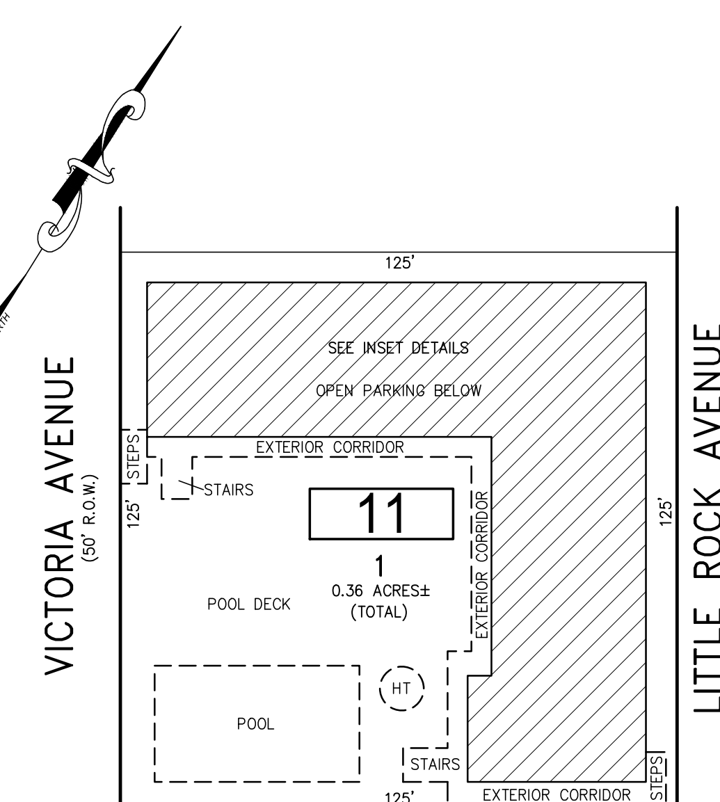
PLAN SCALE: 1"=30'
