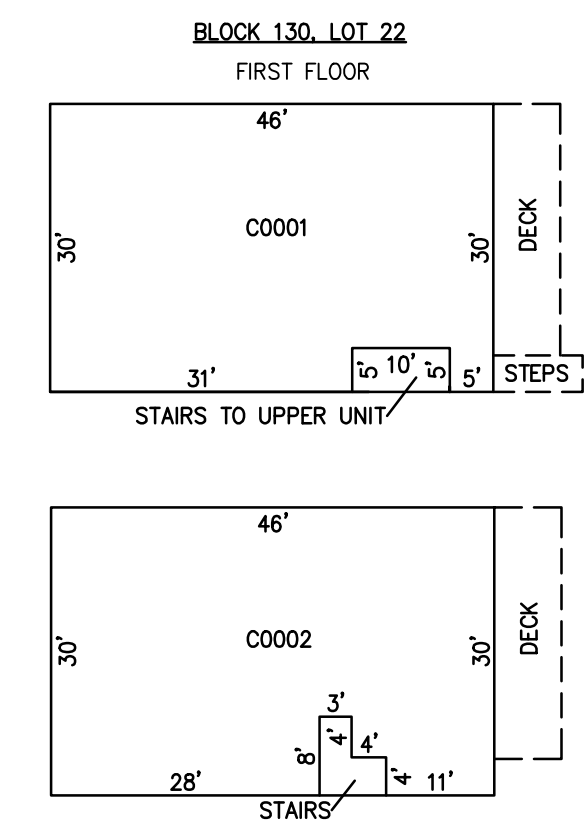
DETAILS SCALE: 1"=20'
