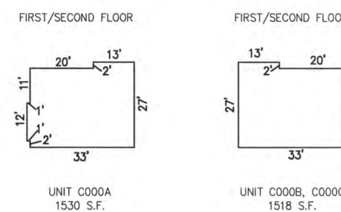
DETAILS SCALE: 1"=30'
