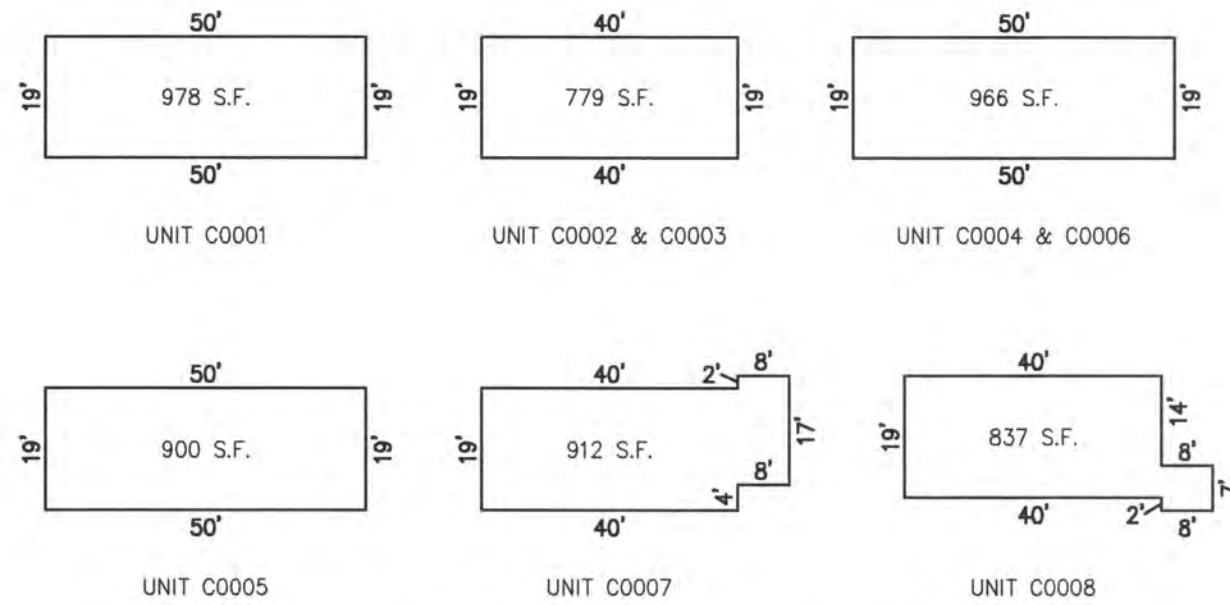
DETAILS SCALE: 1"=30'
